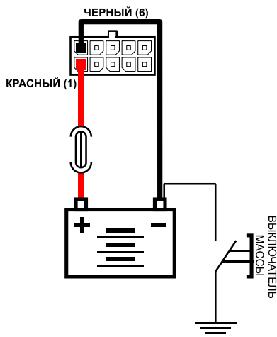
Подключение питания устройства CAN-LOG 2.
